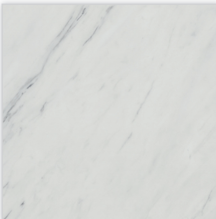
Kolekcja wineo 800 stone XL w wersji bezklejowej Connect, dekor White Marble, symbol DLC00090. Wymiary [mm]: 914,4/457,2/2,5. Wzór: pełna deska, struktura piaskowa, warstwa użytkowa 0,55 mm, klasa użytkowa 23/33/42. Podłoga dostępna również w wersji klejowej.
